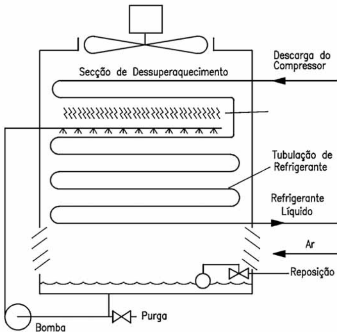
Figura 3.30 - Condensador evaporativo
