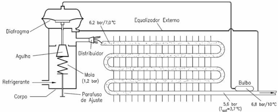
Figura 3.40 - Válvula de expansão termostática de equalização externa
